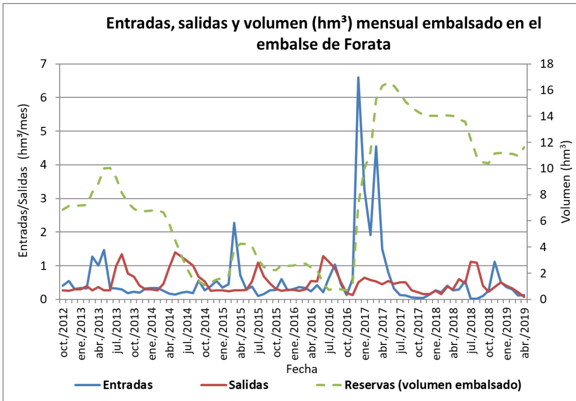
Figura 5 Embalse de Forata: entradas, salidas y volumen mensual embalsado de los últimos años.
